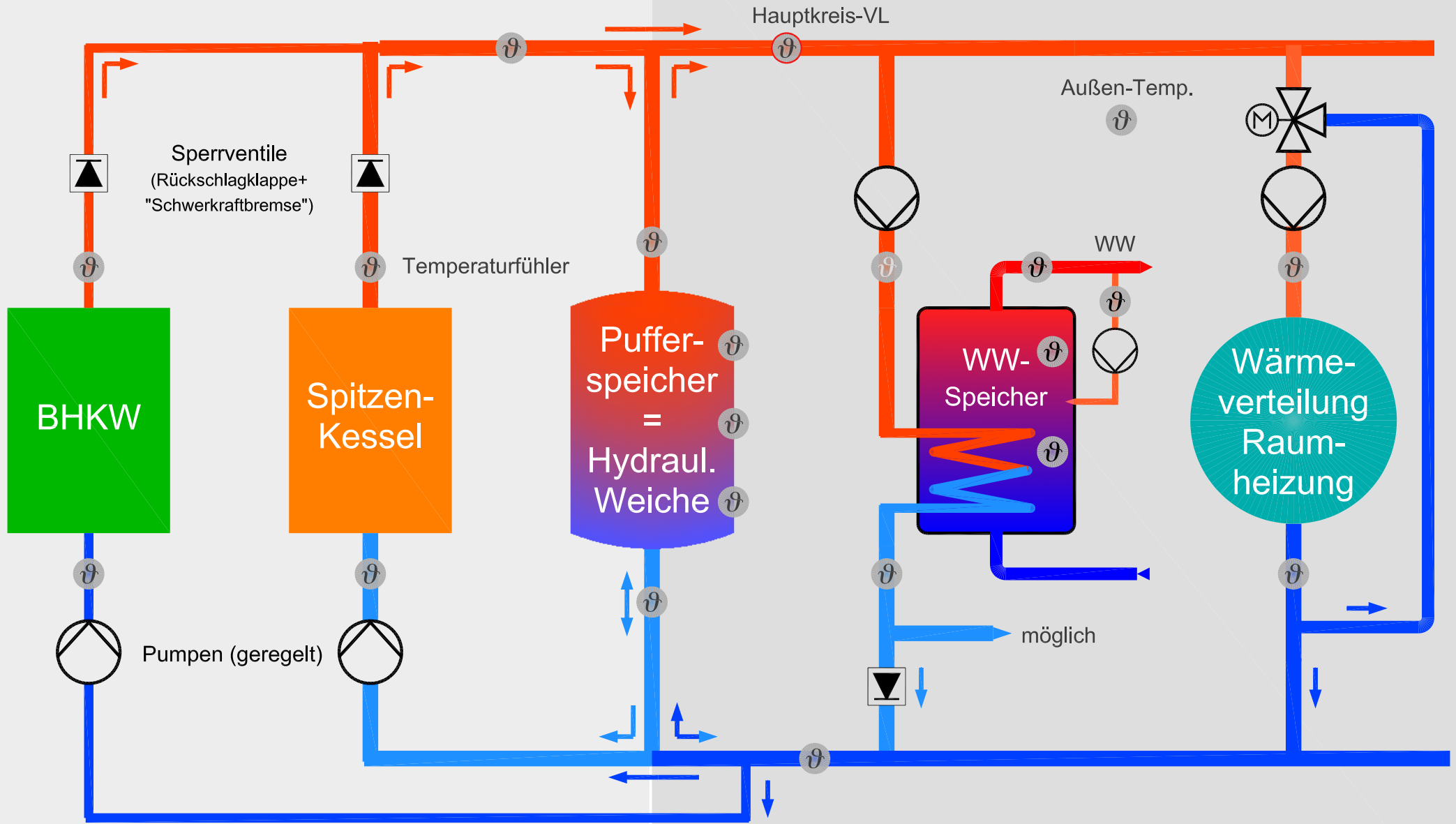
Hydraulik-Variante 1.8 (Puffer als HW + WW-Speicher mit innenl. WT)
