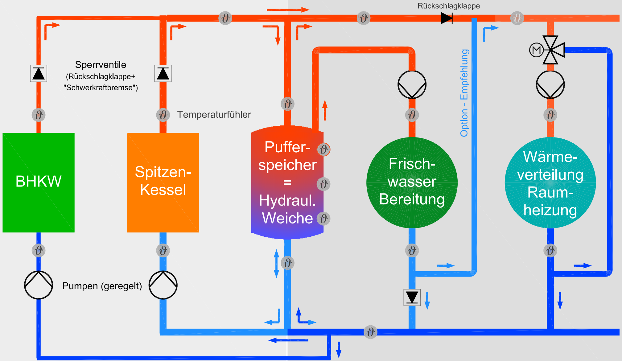
Hydraulik-Empfehlung 1.4 (Puffer als HW + Frischwasserbereitung-1)
