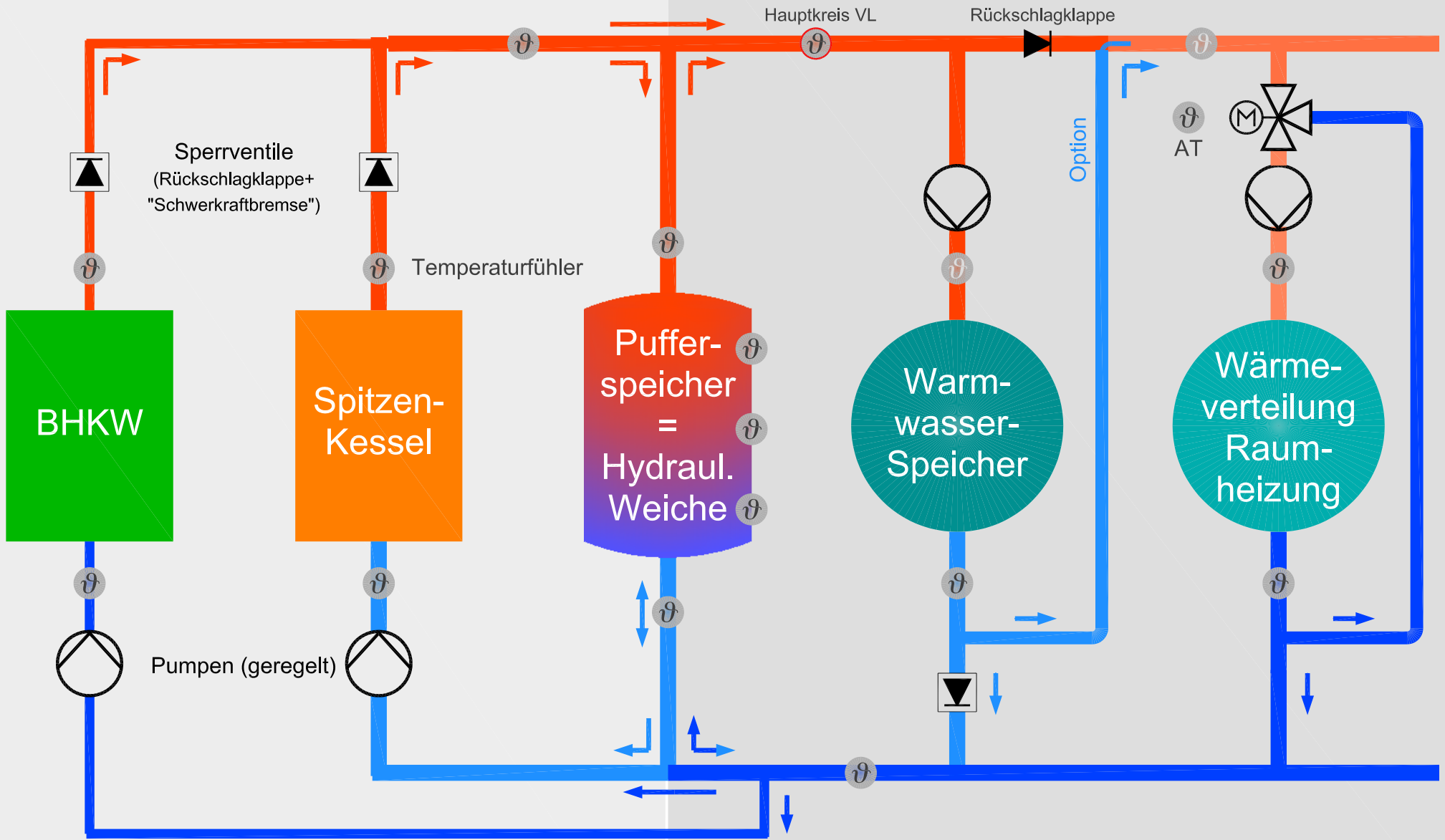
Hydraulik-Empfehlung 1.3 (Pufferspeicher als Hydraulische Weiche, HK-Mischer)
